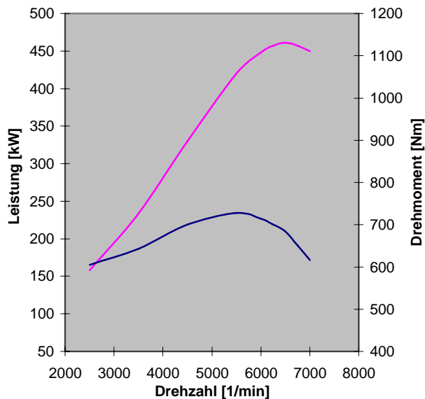
Leistungsdiagramm M297 E69
